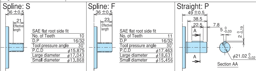
Fig. 1 Shaft end
