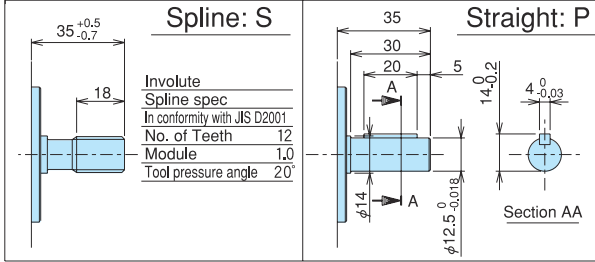
Fig. 1 shaft end
